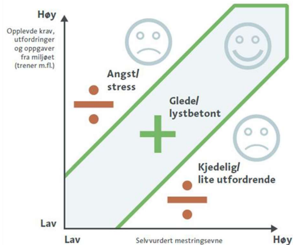
Figur 2: Flytsonemodellen
